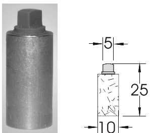
Nr. 2006M Alu M6
