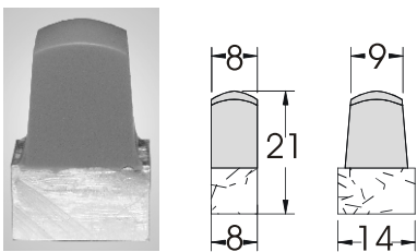
Nr. 2015 Alu M5
