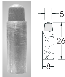
Nr. 363 Alu M4
