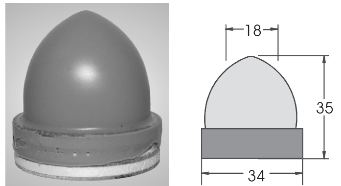
Nr. 97 Nr. 97 Alu M6 H 35
