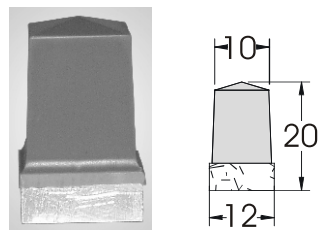
Nr. 2003 Alu M6
