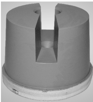
S Ø64 H 59 Innenloch Ø21
