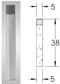
Nr. 197 Alu M5
