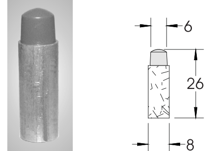
Nr. 2195 Alu M6
