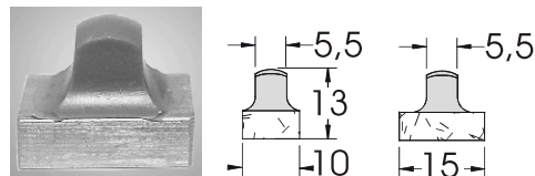
Nr. 2008M Alu M6
