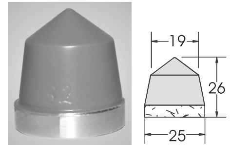
Nr. 32 Alu M6
