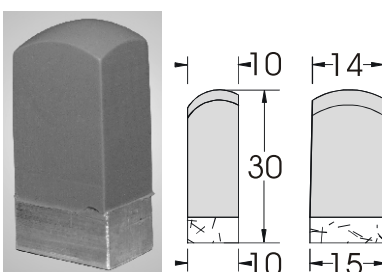
Nr. 2015 Alu M5
