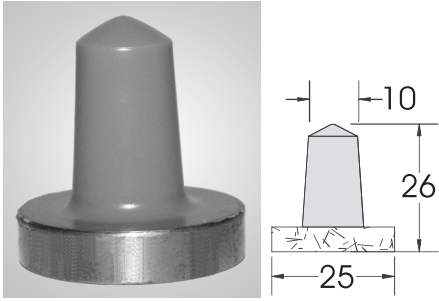
Nr. 579 Alu M5
