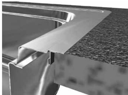
SlimTop: Die Spüle oder das Becken liegt mit einem flachen Rand in der Materialstärke auf der Arbeitsplatte auf.
