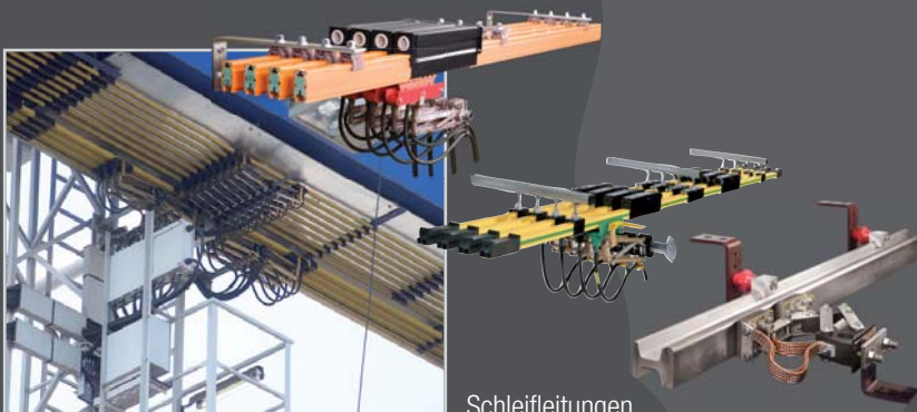
Schleifleitungen
