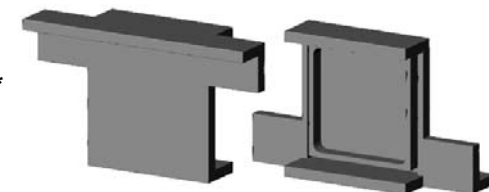
Abschlussstopfen für quadratisches Sonderprofil 50x50 mm mit Stegen* End plug for special square profile 50x50 mm with wings* Embout à insérer pour profil carré spécial 50x50 mm avec des appuis*
