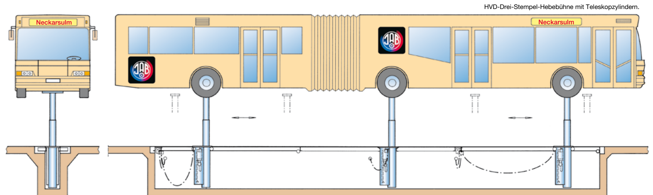
HVD-Drei-Stempel-Hebebühne mit Teleskopzylindern.
